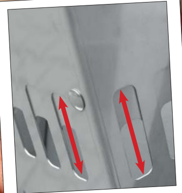
Verstellmöglichkeit Flexblech
